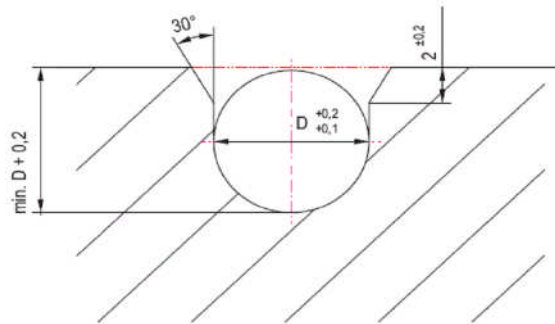
Nut-Abmessung RHEflex rund
